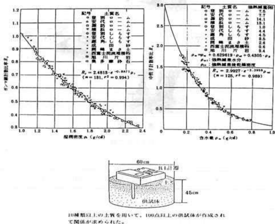
図－３ 計数率比と湿潤密度および含水量の検定例 (地盤工学会「地盤調査法」から引用)
