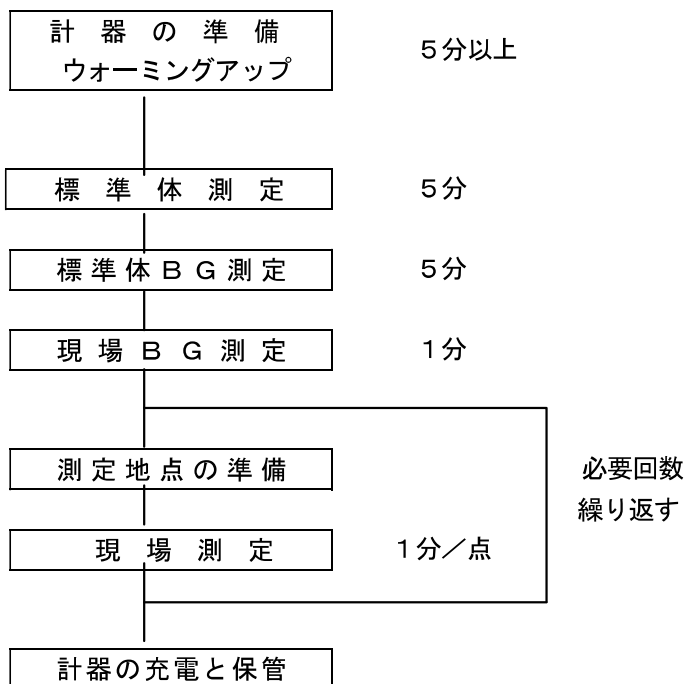
図－5 測定の手順の例
