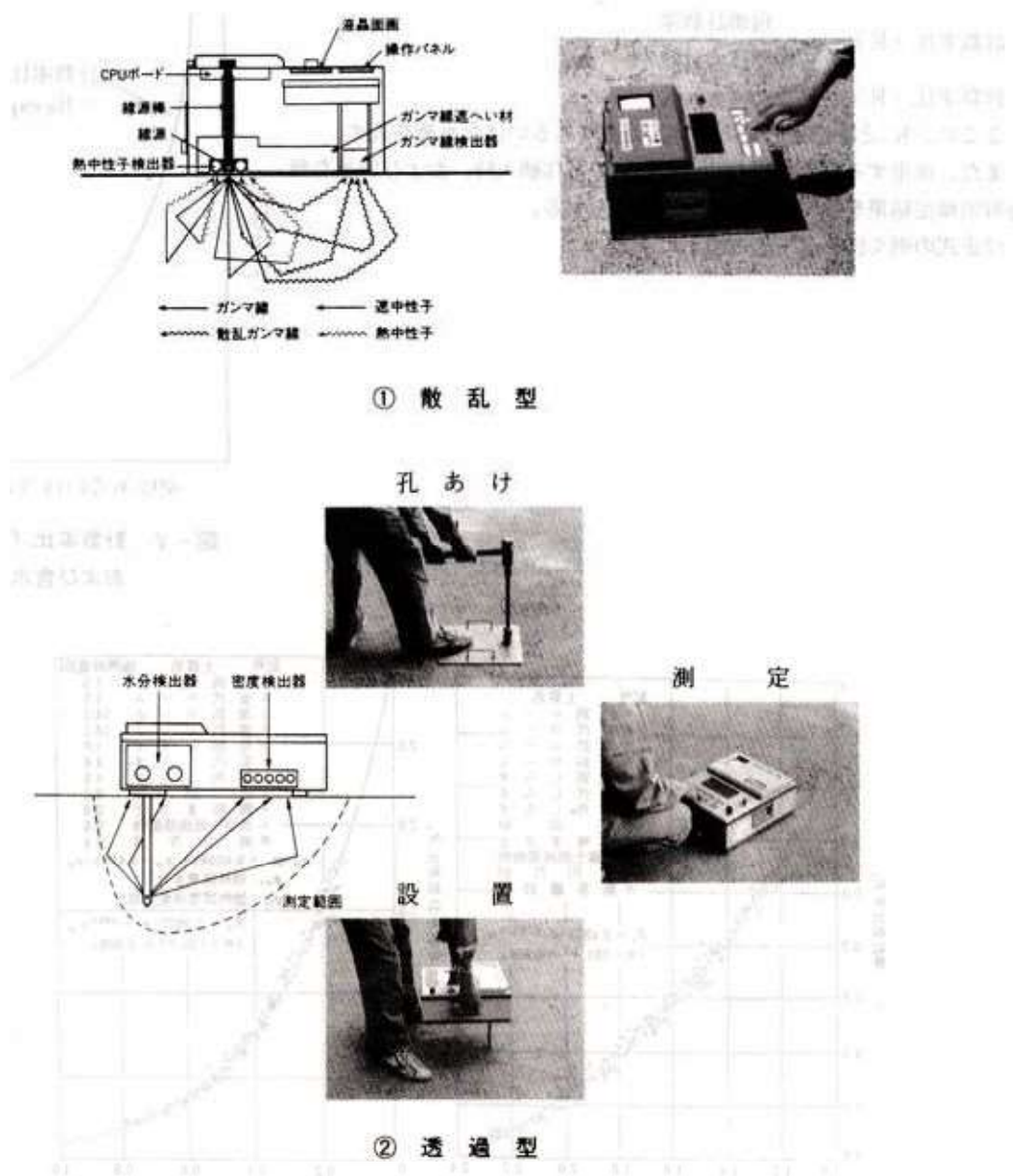
図ー１ R I 計器の概要
