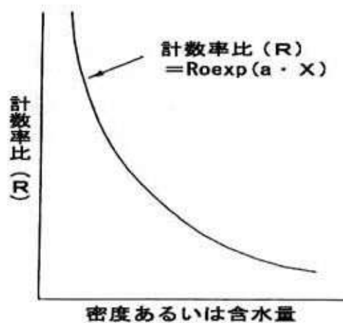
図－２ 計数率比 (R) と密度および含水量の関係
