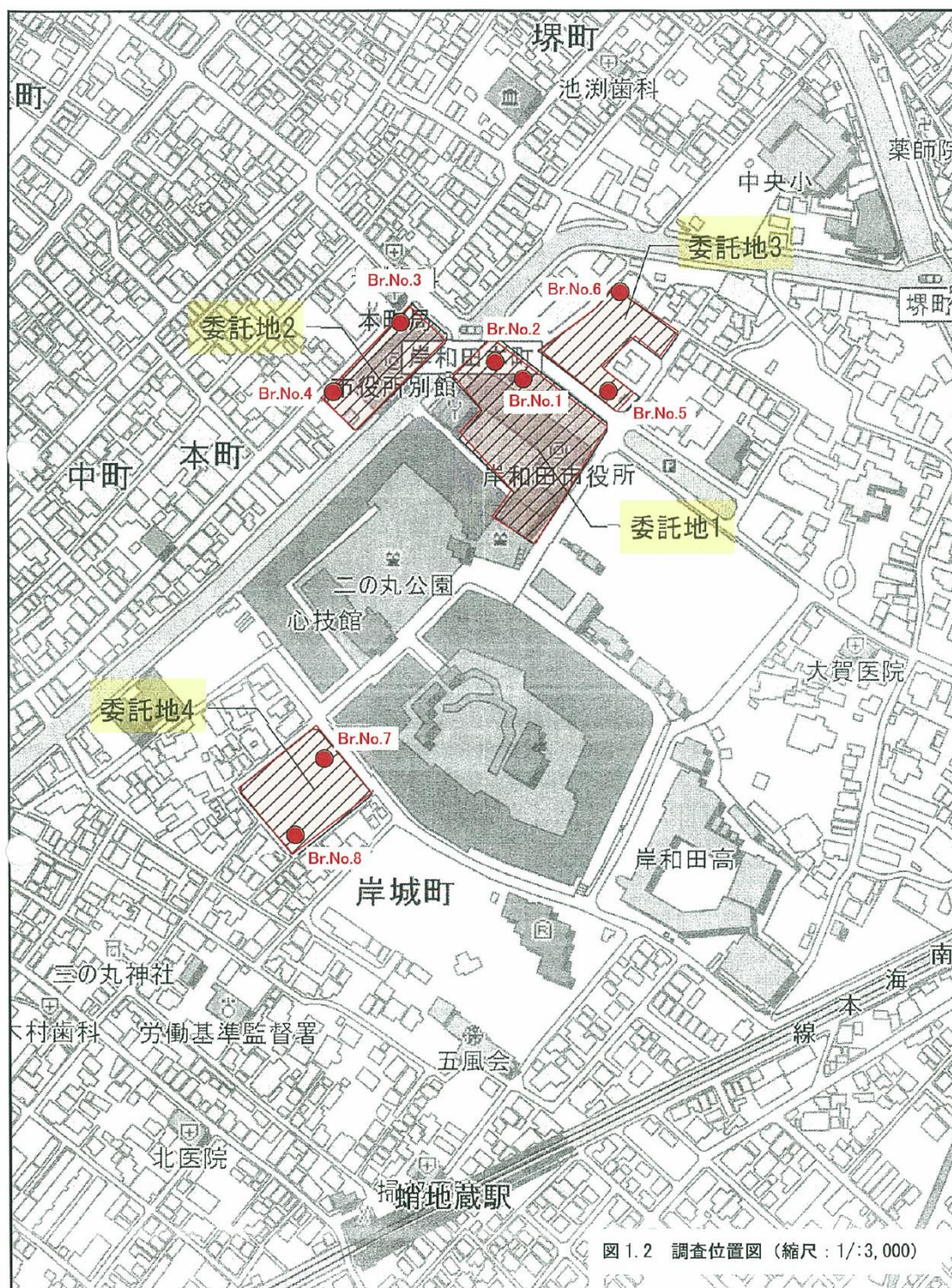
図 3-7 対象敷地とボーリング位置図
