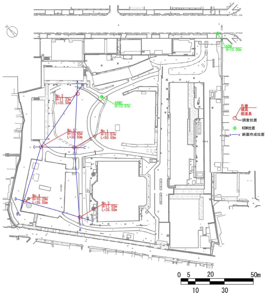
図 3-7 対象敷地とボーリング位置図
