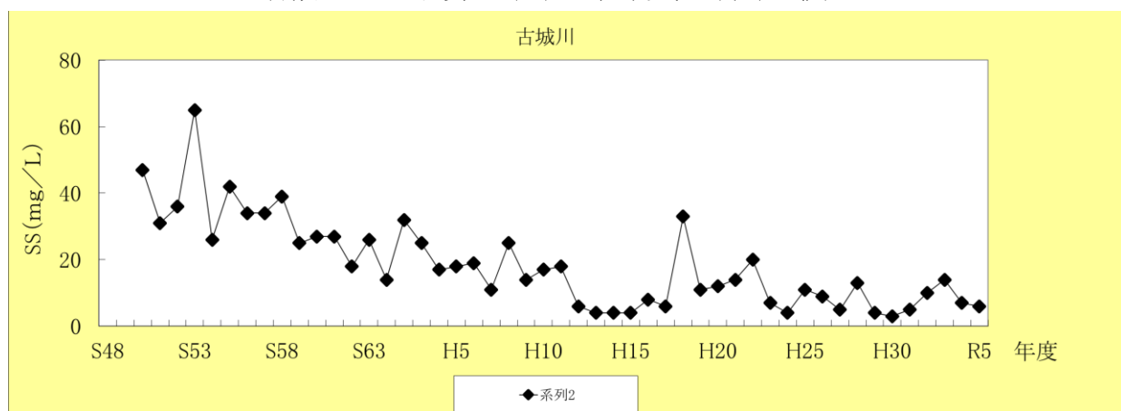
古城川 浮遊物質量 (SS) の経年変化 (年平均値)
