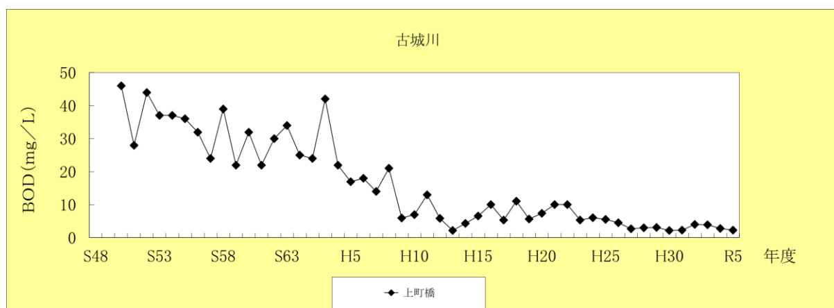
古城川 生物化学的酸素要求量（BOD）の経年変化（年平均值）
