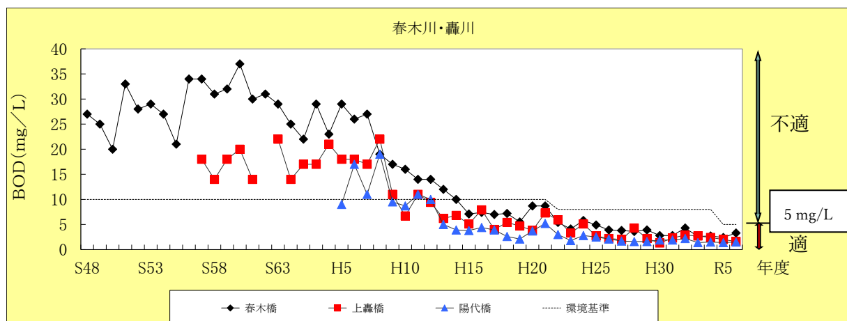
春木川、轟川 生物化学的酸素要求量 (BOD) の経年変化 (75%値)
