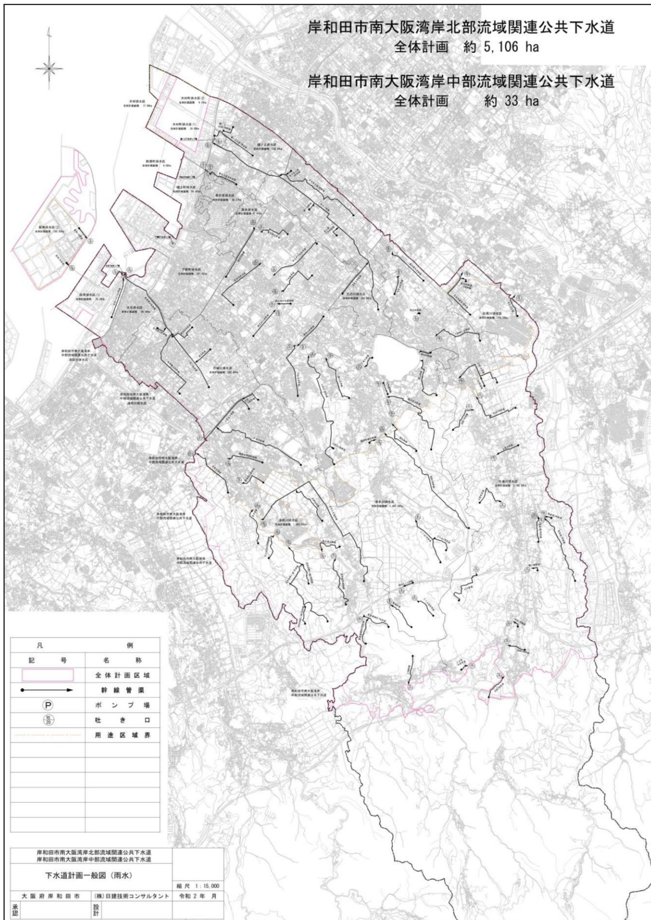
図 2 岸和田市下水道計画図(雨水)
