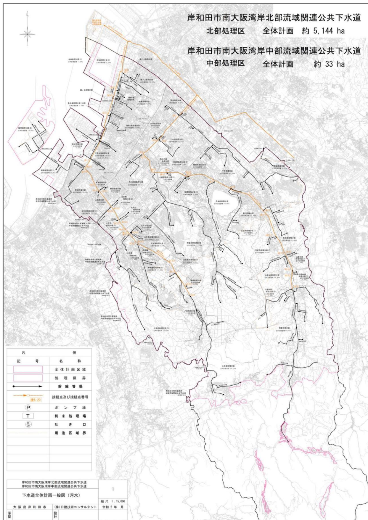
図 1 岸和田市下水道計画図（汚水）
