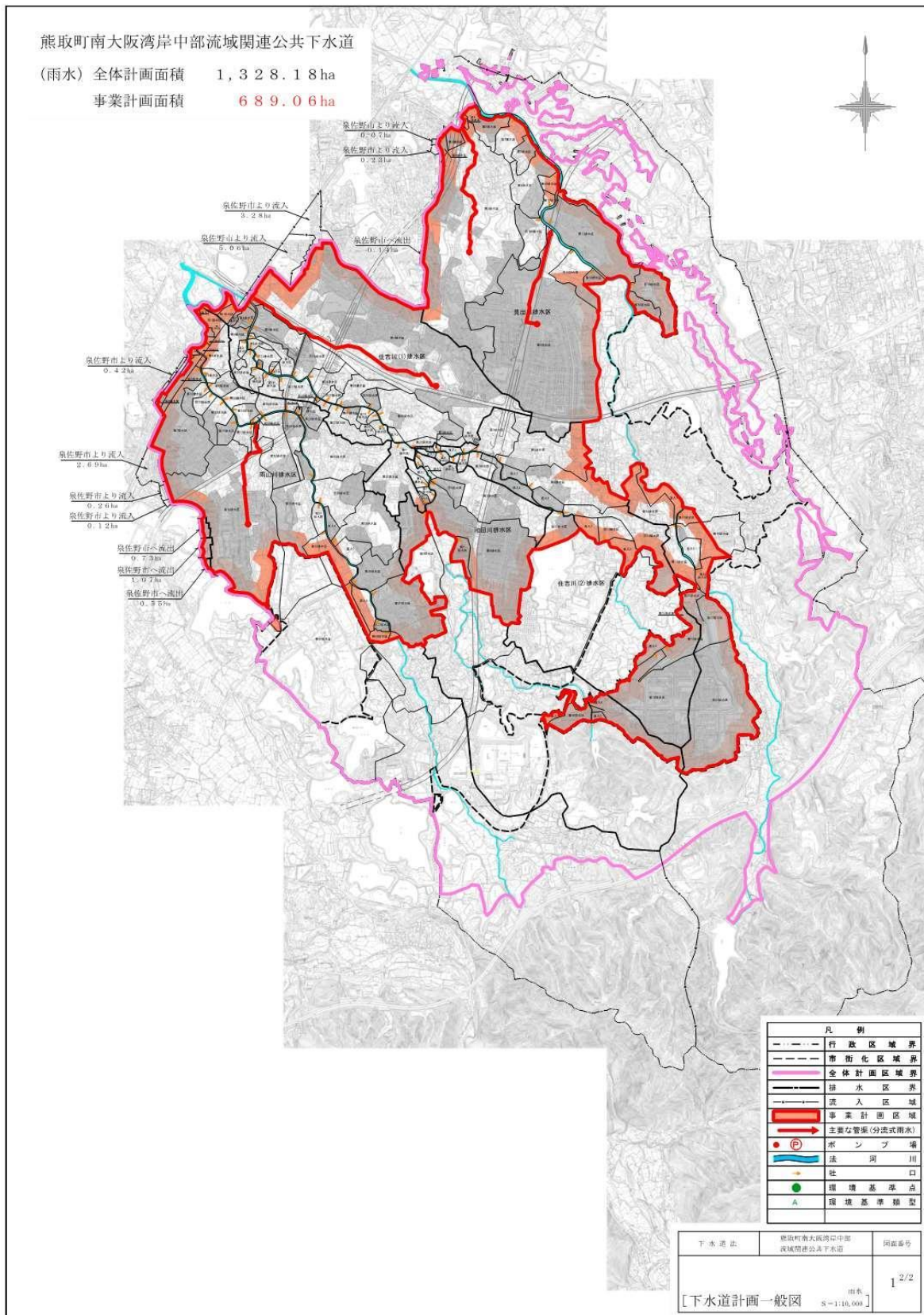
図 6-2 下水道全体計画図(雨水)
