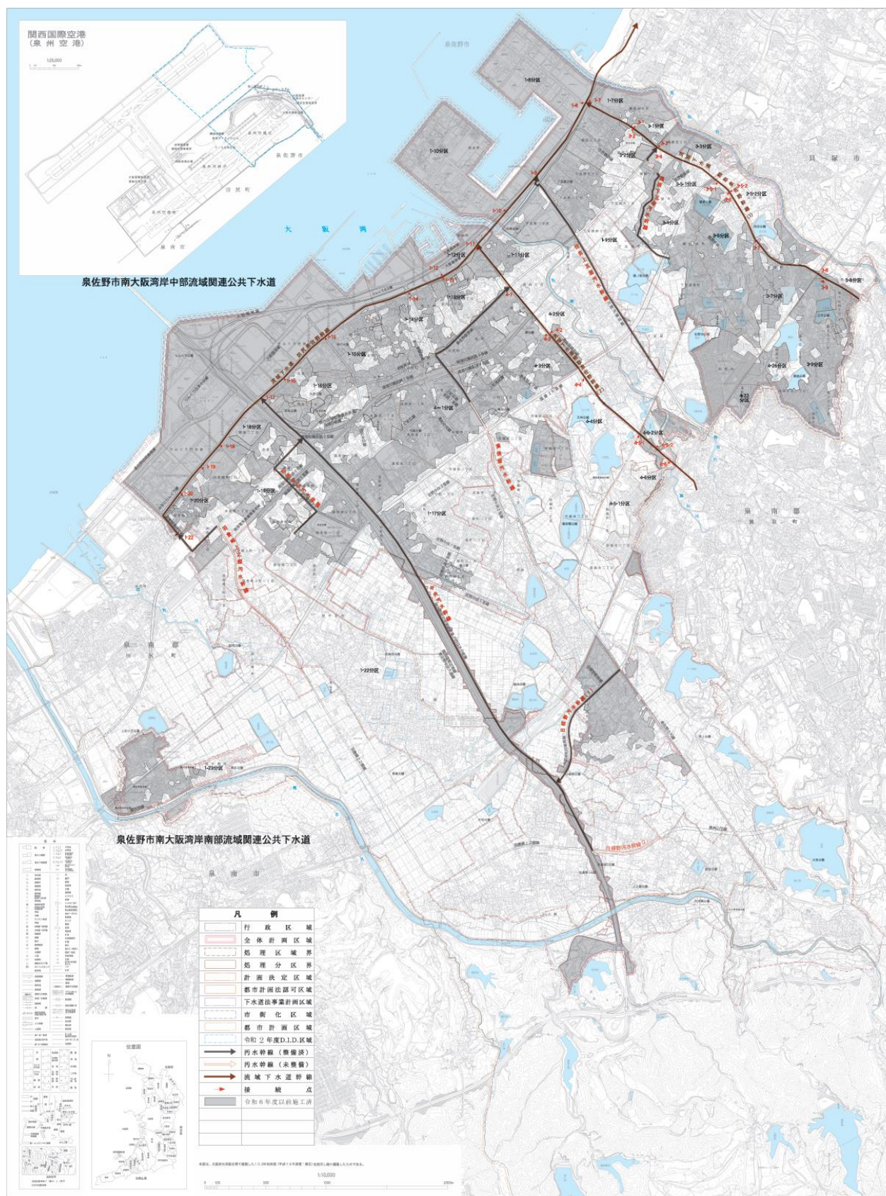
図 4-1 下水道全体計画図（污水）
