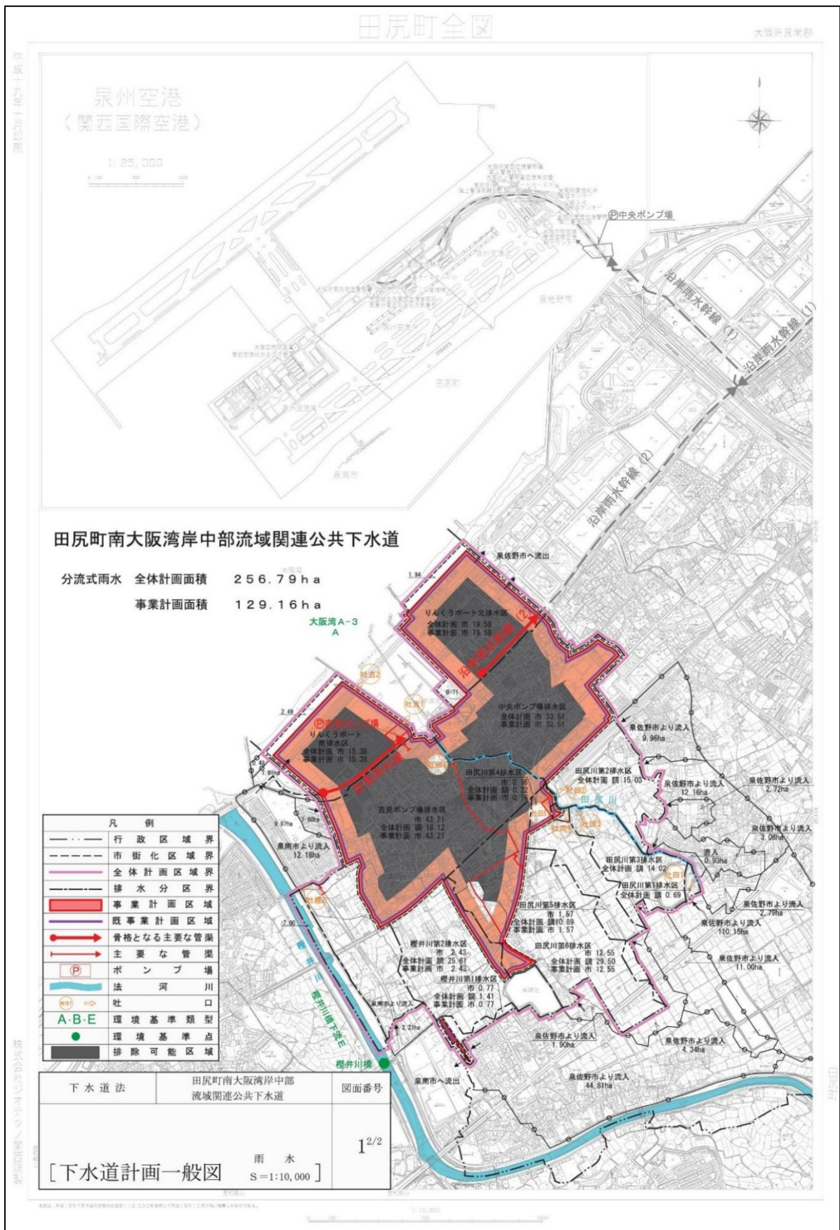
図 5-2 下水道事業計画図（雨水）
